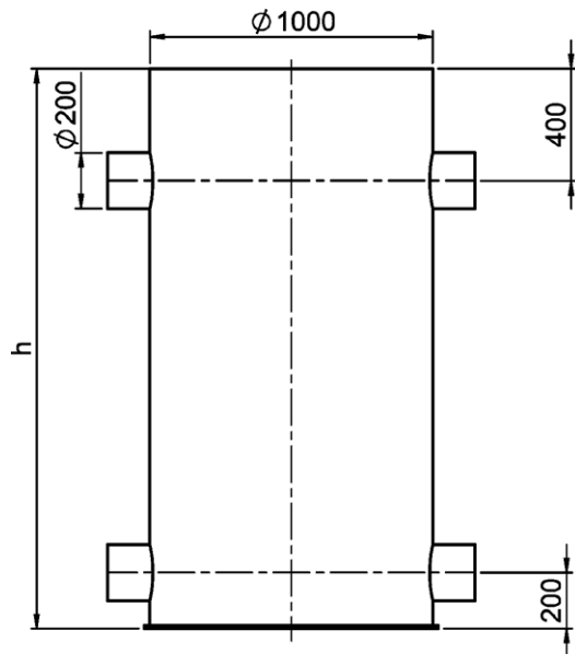
Artikel Nr. 310061020 / 310061030 (Behälter 1500 L / 2300 L)
