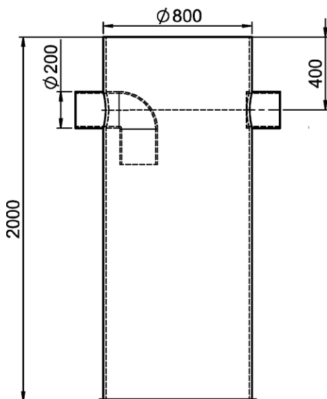
Artikel Nr. 310070820 (Grobfang 800 L)
